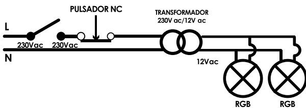
INSTALACIÓN PARA SINCRONIZADOR MEDIANTE PULSADOR EXTERNO. (539128)
