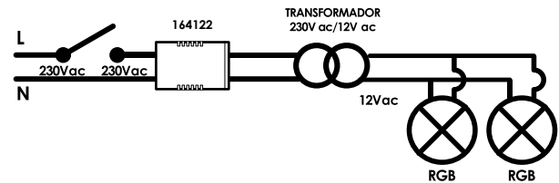
INSTALACIÓN PARA SINCRONIZADOR WIRELESS. (539128)
