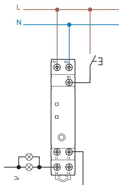
Tipo 12.C1 Botão pulsador B1 ligado na fase
